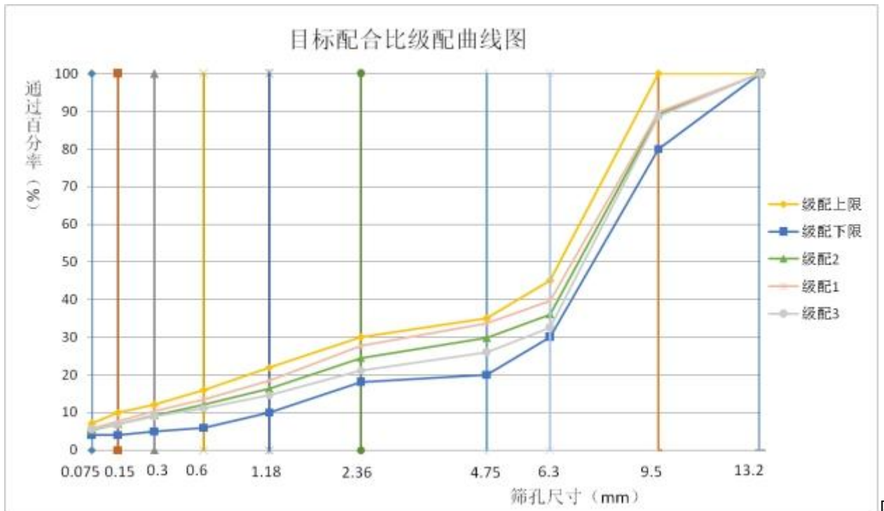
A.1 级配曲线
