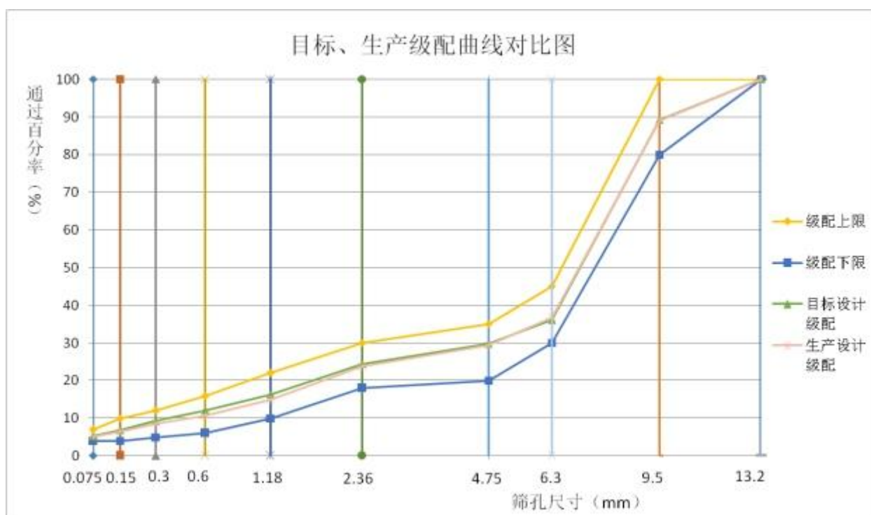
图A.2 目标、生产配合比级配曲线对比图
