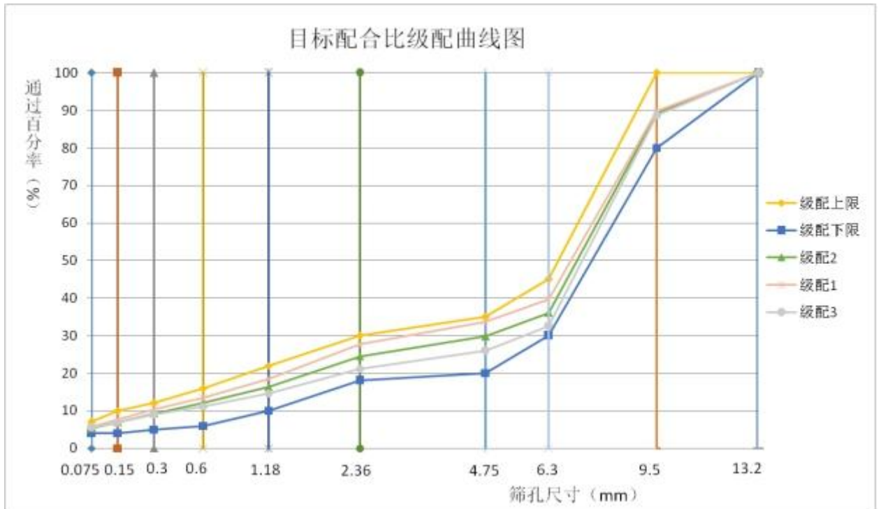
图 A.1 级配曲线
