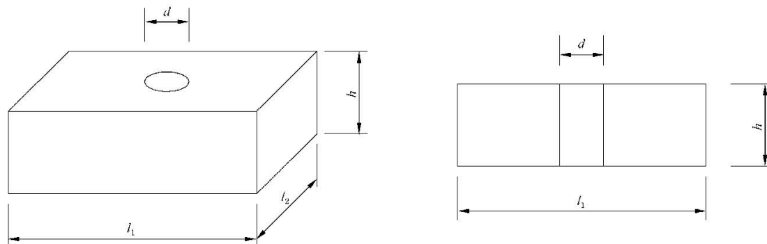
图 1 带竖孔内置箱体成孔芯模
